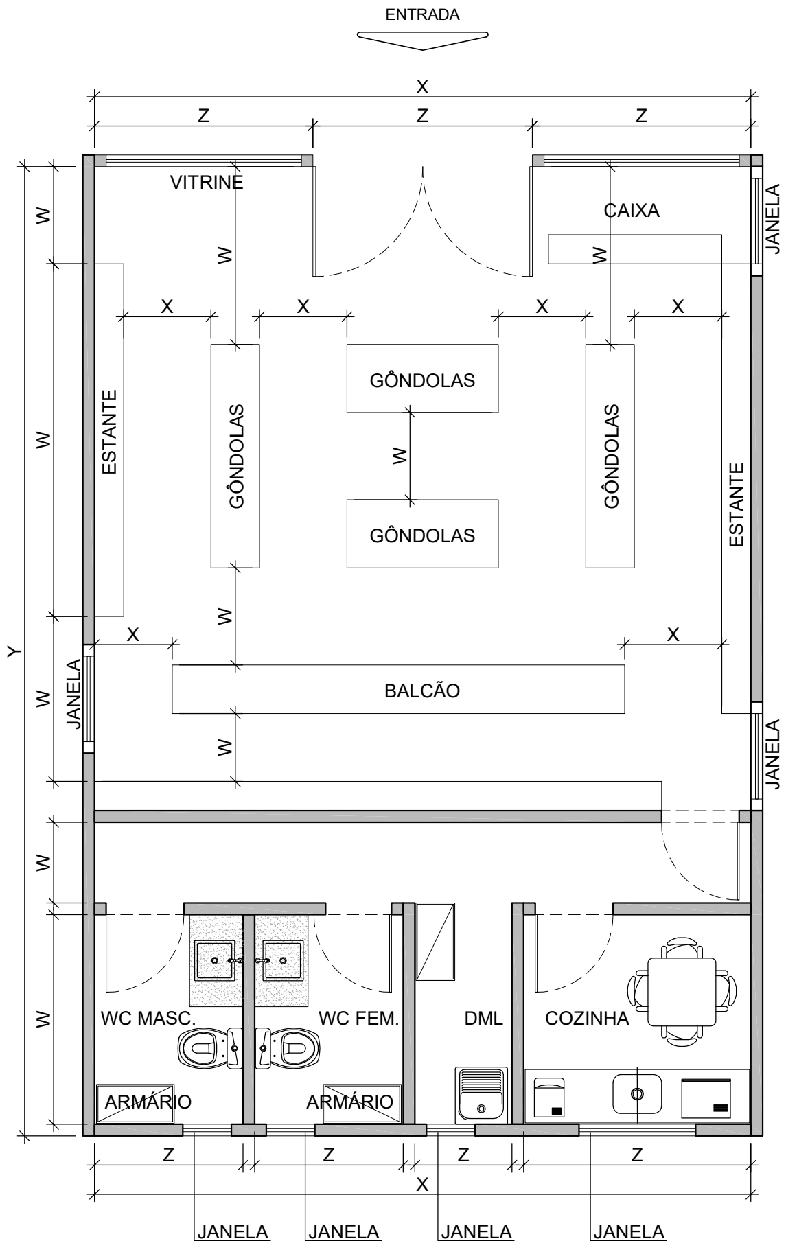
CROQUI - PLANTA BAIXA SEM ESCALA
